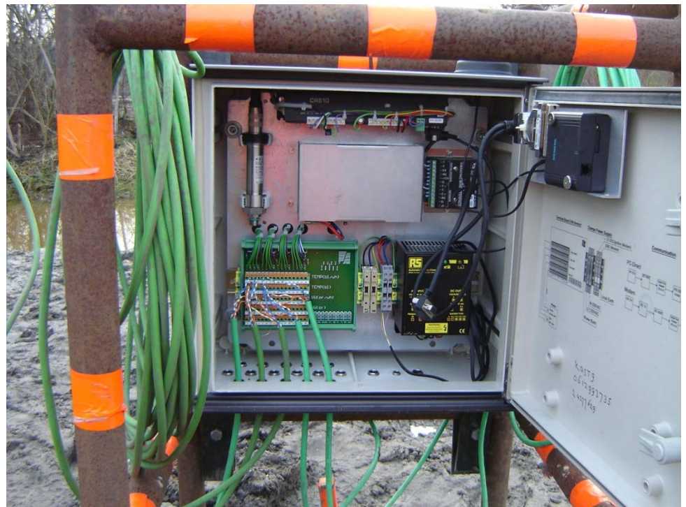
Controle wateroverspanning bij ophoging.
