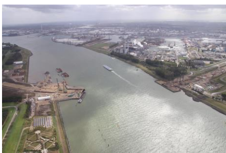
Foto's: Luchtfoto Maasdelatunnel, afzinken element Limfjordtunnel eind jaren 60, transport caisson voor Çannakale brug
