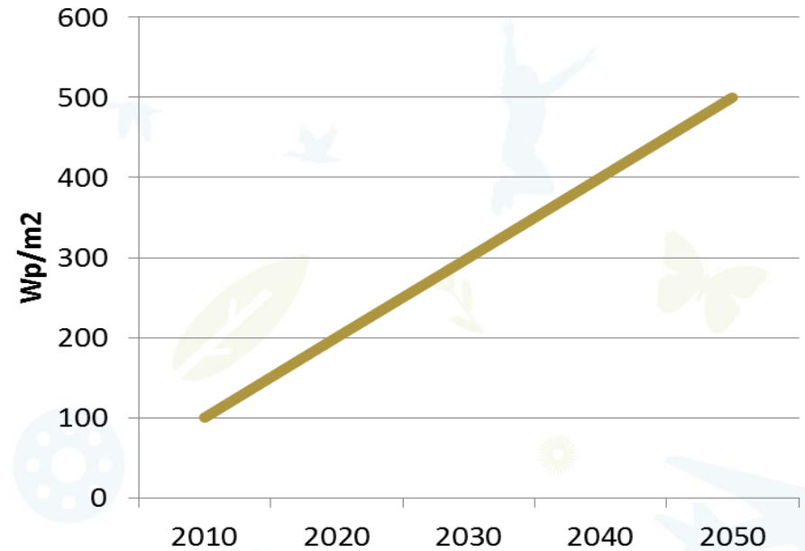
Ontwikkeling rendement PV-panelen
