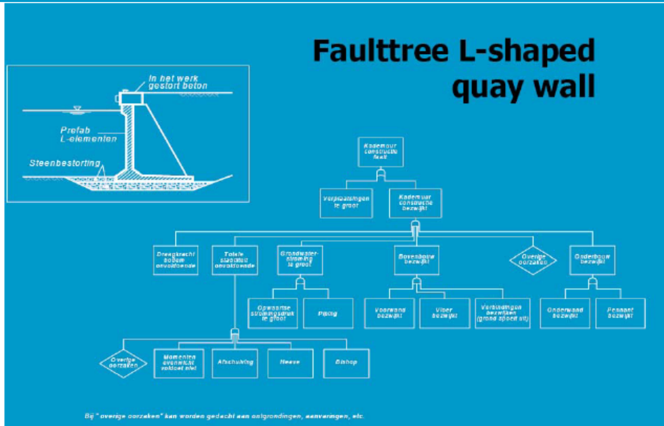
Figuur 2: Foutenboom L-vormige kademuur
